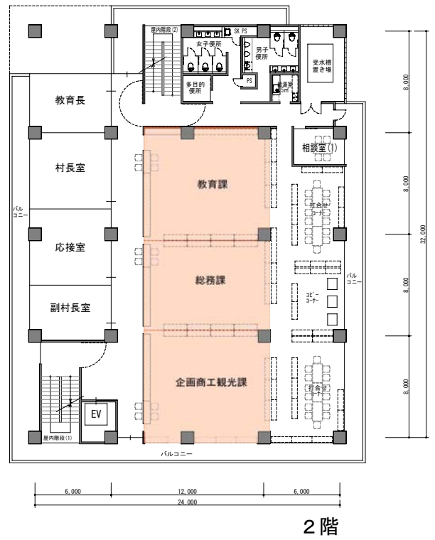
国頭村新庁舎平面レイアウト図 Scale : 1/200
